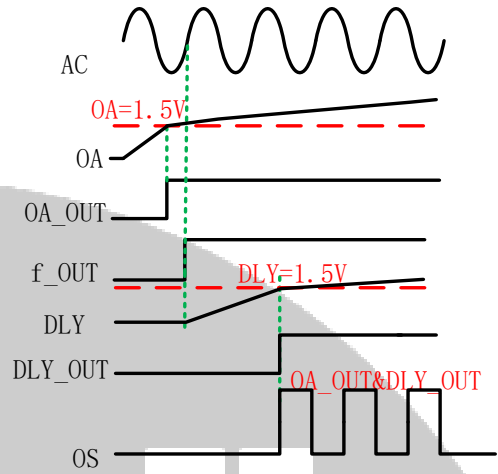
Figure 6. 工作原理图
