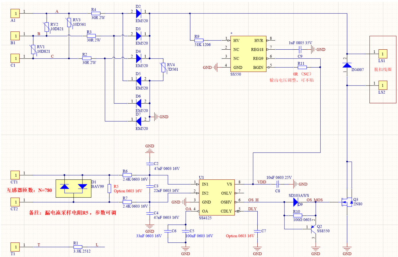
Figure 10. SS4125B 三相下进线应用
