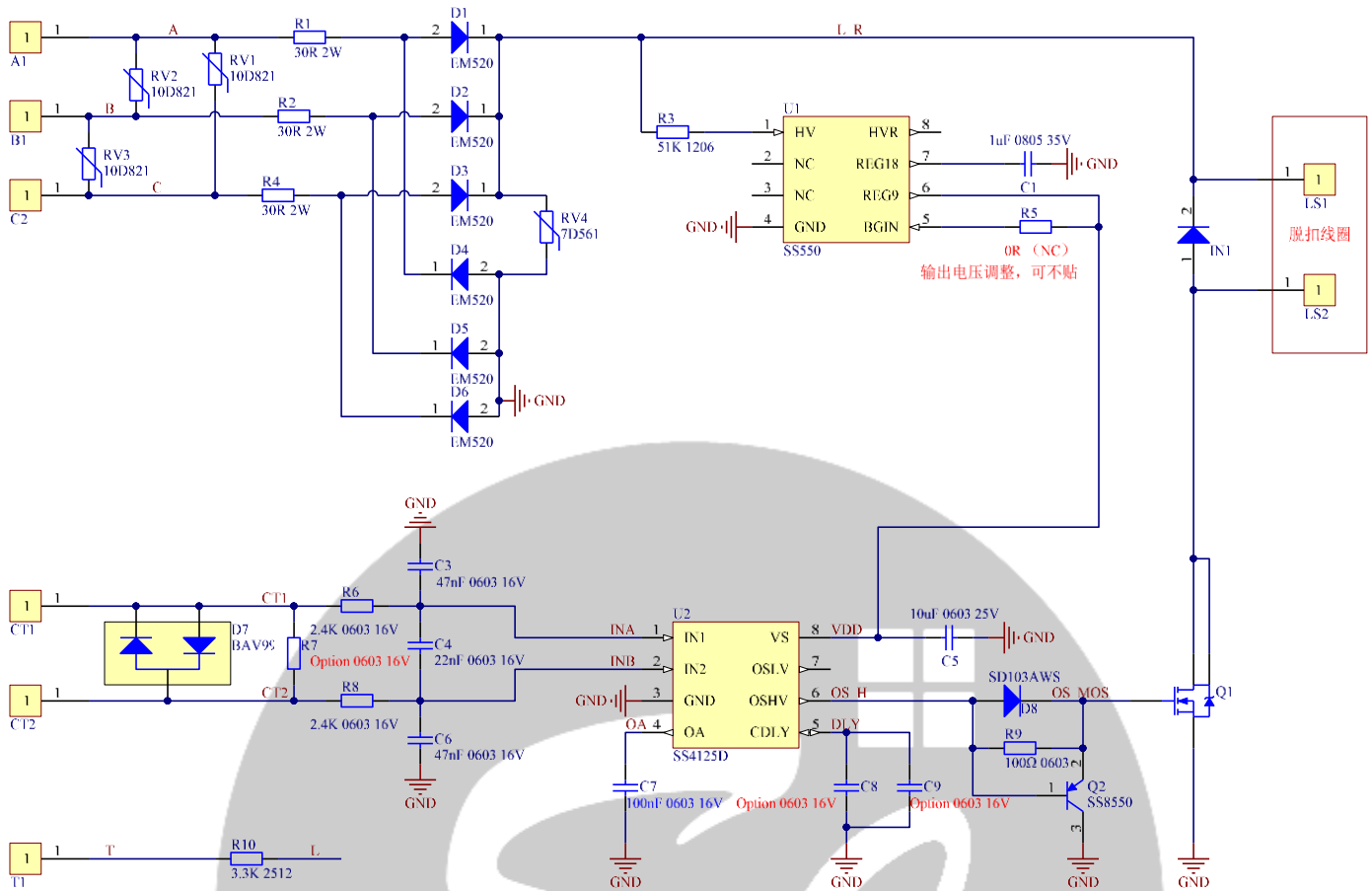
Figure 10. SS4125D 三相上、下进线应用典型电路
