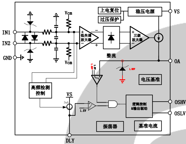
Figure 5. 芯片内部框图
