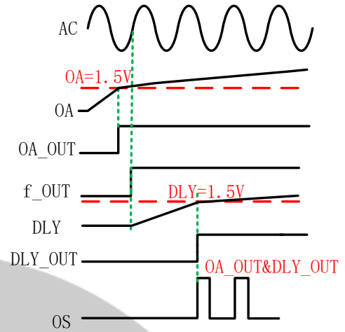
Figure 6. 工作原理图
